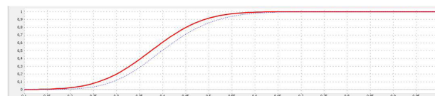
Curva con una variazione molto debole di lift-off.
