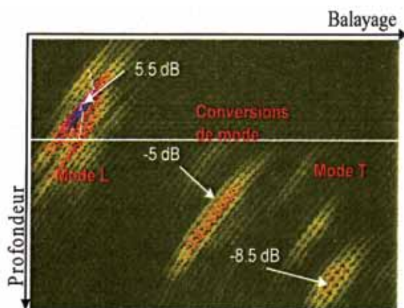
BScan issu de l'inspection. Plusieurs échos et une proposition de diagnostic, défaut proposé est dessiné.
