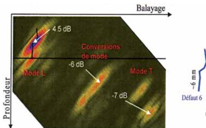
Simulation réalisée à partir du diagnostic proposé. Bonne corrélation des échos obtenus.
