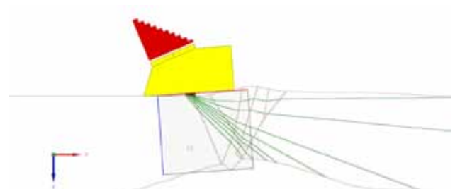
Sensor posicionado sobre a soldadura, influencia dos materiais da soldadura sobre o traçado de raio.
