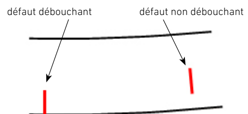
Pièce comportant deux défauts en paroi externe : débouchant et non débouchant.
