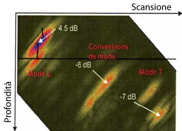
Simulazione realizzata a partire dalla diagnosi proposta. Buona correlazione degli eco ottenuti.
