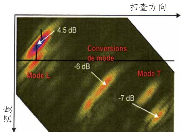
该图是根据裂纹形状做的CIVA仿真的B扫视图。仿真结果与实验结果可以很好的对应,从而验证了裂纹的形状。
