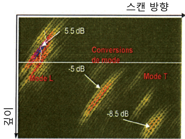
다양한 에코를 보여주는 B-스캔 실험영상. 에코 명칭(label)은 결함의 모양이 아래와 같다고 가정하고 해석하였습니다.
